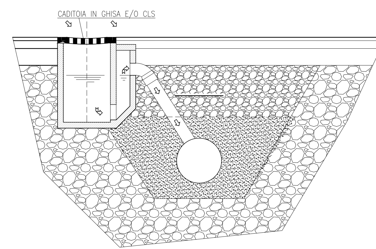
PARTICOLARE CAMERETTA INTERRATA ACQUE BIANCHE/NERE scala 1:20
