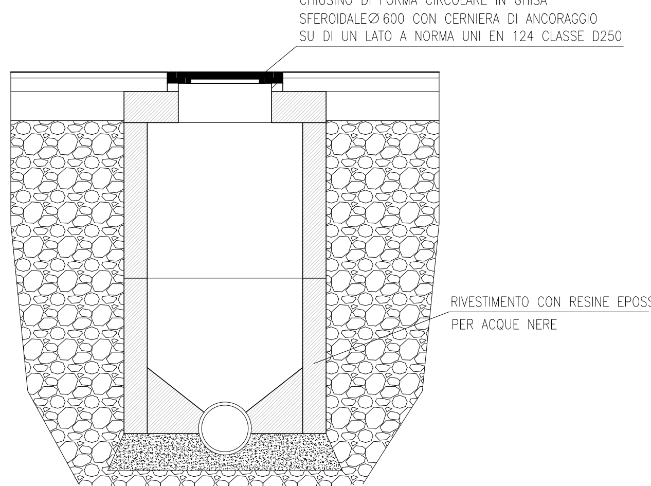
PARTICOLARE CAMERETTA INTERRATA ACQUE BIANCHE/NERE scala 1:20
